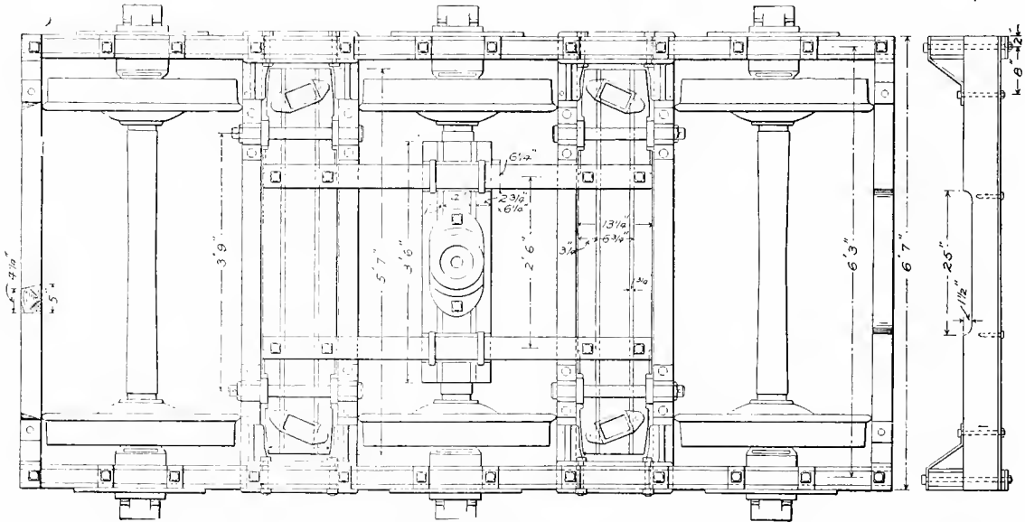
Fig. 4787. Plan.
